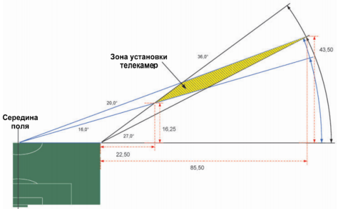
Схема розміщення телевізійних камер офіційного мовника уздовж бічної лінії поля з розрахунком згідно рекомендацій UEFA
